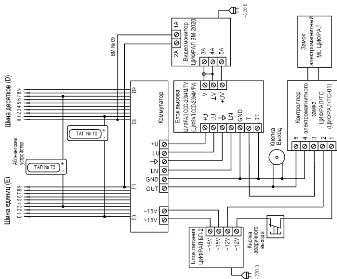
Рисунок В.2 Схема подключения домофонов ЦИФРАЛ ССД-2094М/TV, ЦИФРАЛ ССД-2094М/PV (для вариантов исполнения «VC» использовать видеомонитор ЦИФРАЛ ВМ-3020)
