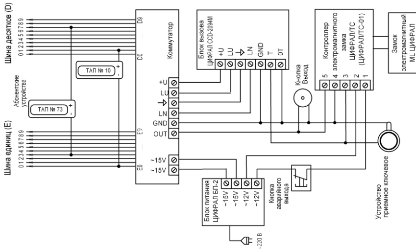
Рисунок В.1 Схема подключения домофона ЦИФРАЛ CCD-2094М
