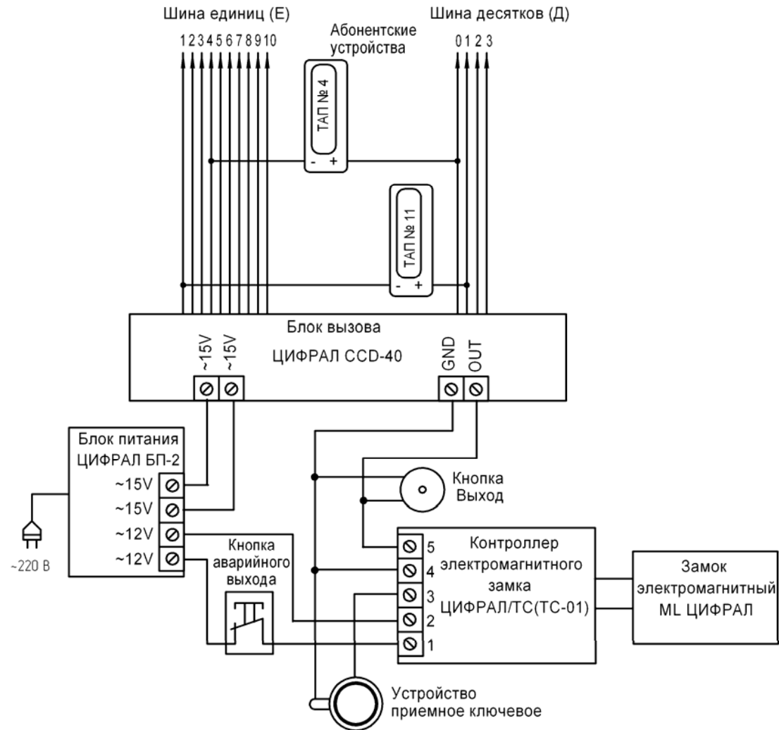
Рисунок Б.1 Схема подключения домофона ЦИФРАЛ ССД-40
