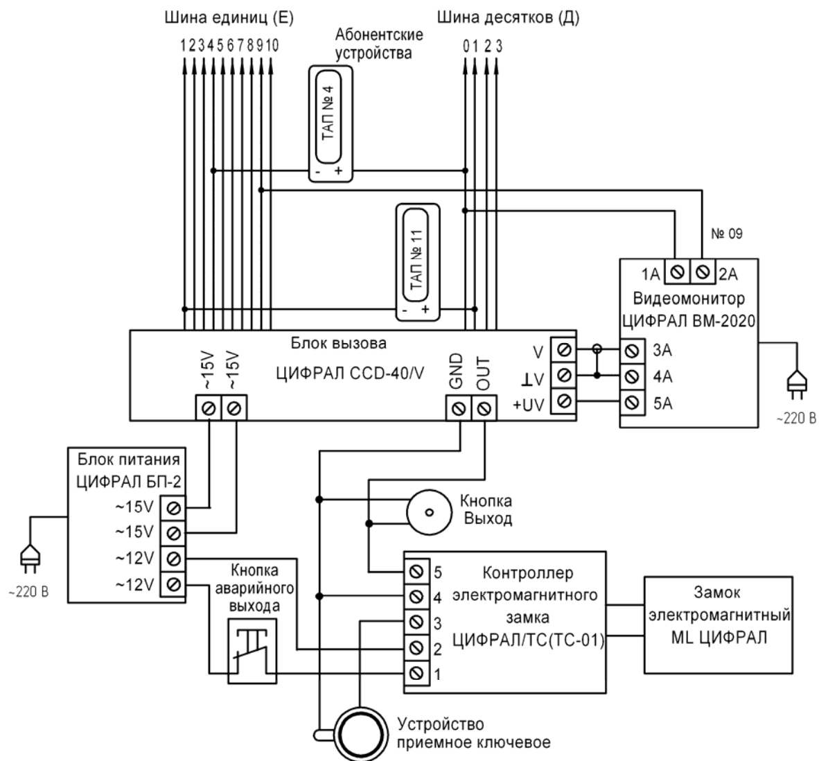
Рисунок Б.2 Схема подключения домофона ЦИФРАЛ ССД-40/V (для варианта исполнения «VС» использовать видеомонитор ЦИФРАЛ ВМ-3020)
