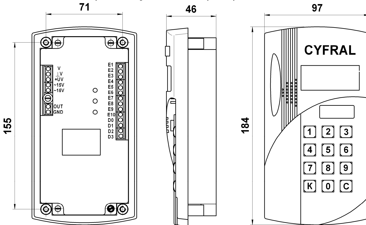
Рисунок А.1 Габаритные и установочные размеры блоков вызова ЦИФРАЛ ССД-40, ЦИФРАЛ ССД-40/У, ЦИФРАЛ ССД-40/УС
