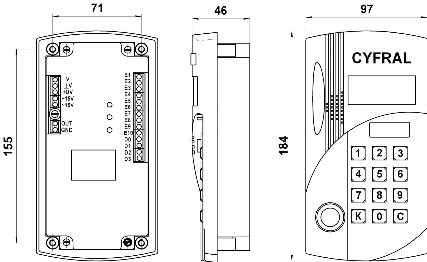
Рисунок А.1 Габаритные и установочные размеры блоков вызова ЦИФРАЛ ССД-40/ТС, ЦИФРАЛ ССД-40/ТСV, ЦИФРАЛ ССД-40/ТСVС, ЦИФРАЛ ССД-40/Р, ЦИФРАЛ ССД-40/РV, ЦИФРАЛ ССД-40/РVС
