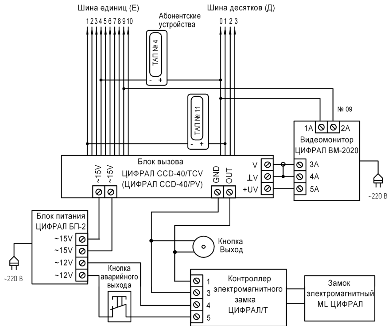
Рисунок Б.4 Схема подключения домофонов ЦИФРАЛ CCD-40/ТСV, ЦИФРАЛ CCD-40/PV (для варианта исполнения «VС» использовать видеомонитор ЦИФРАЛ ВМ-3020)
